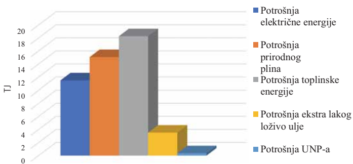
Slika 1 Struktura energenata u neposrednoj potrošnji energije u sektoru zgrada u vlasništvu i korištenju Grada Velike Gorice za 2017. godinu (Izvor: Informacijski sustav za gospodarenje energijom, ISGE)
